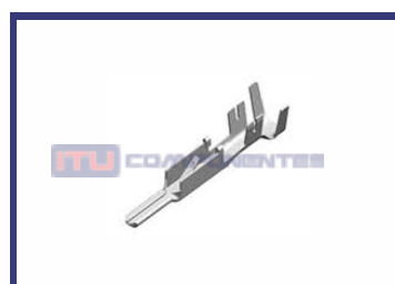
Terminal Macho Metri Pack cabo de 2,5 a 5,0 mm Série 280 Cód.: 3287
