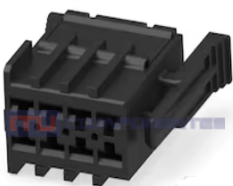
Conector 8 vias Fêmea JPT Cód.: 1405
